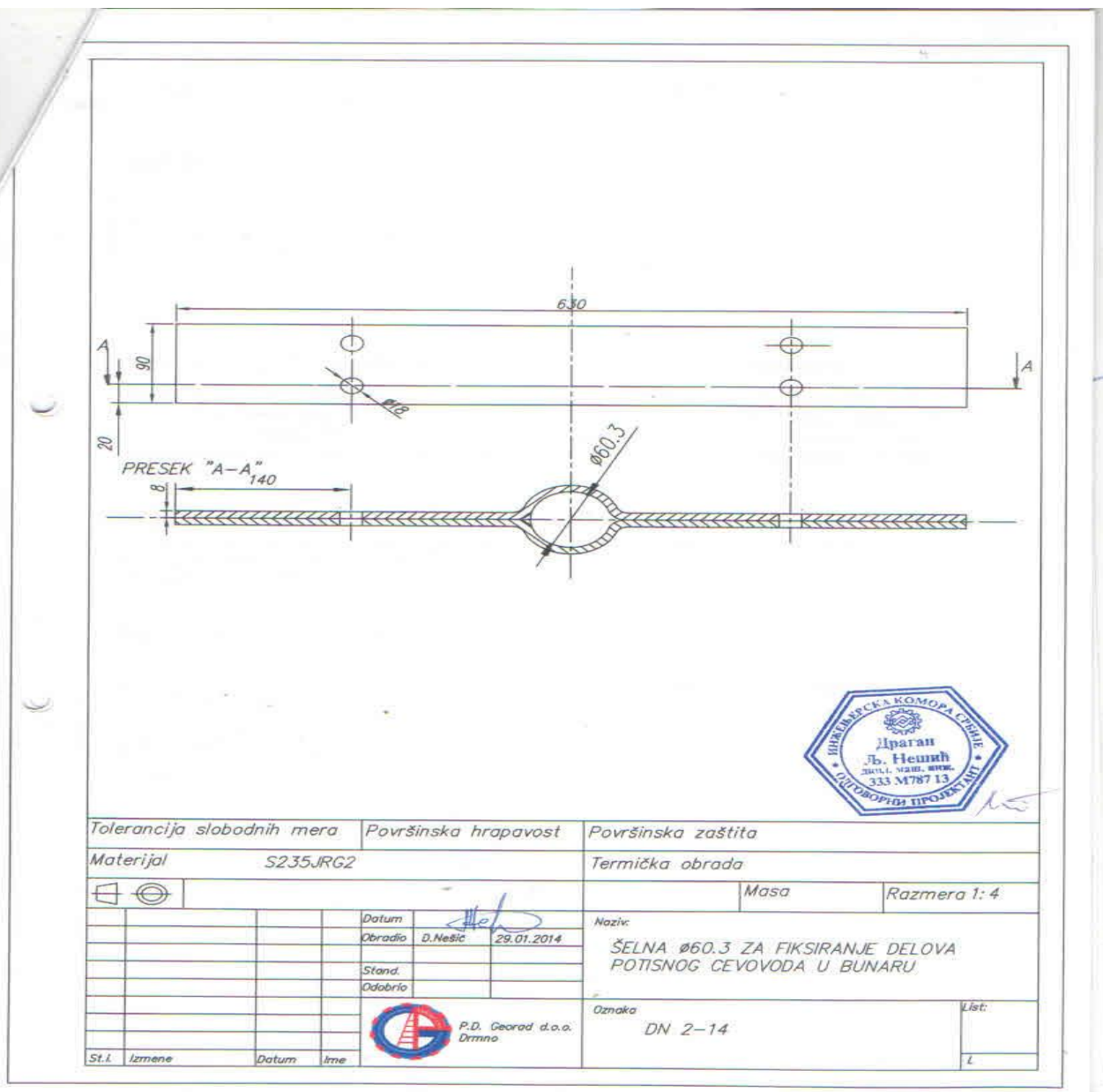
Цртеж бр.2 , Челични носач потисног цевовода-шелна позиције 48-51 на тех. спецификацији
