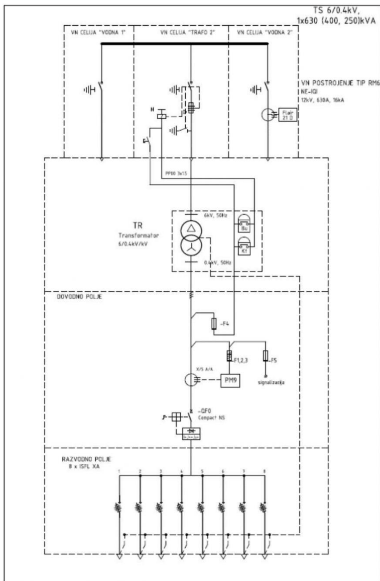
Слика 40:Једнополна шема ТС
