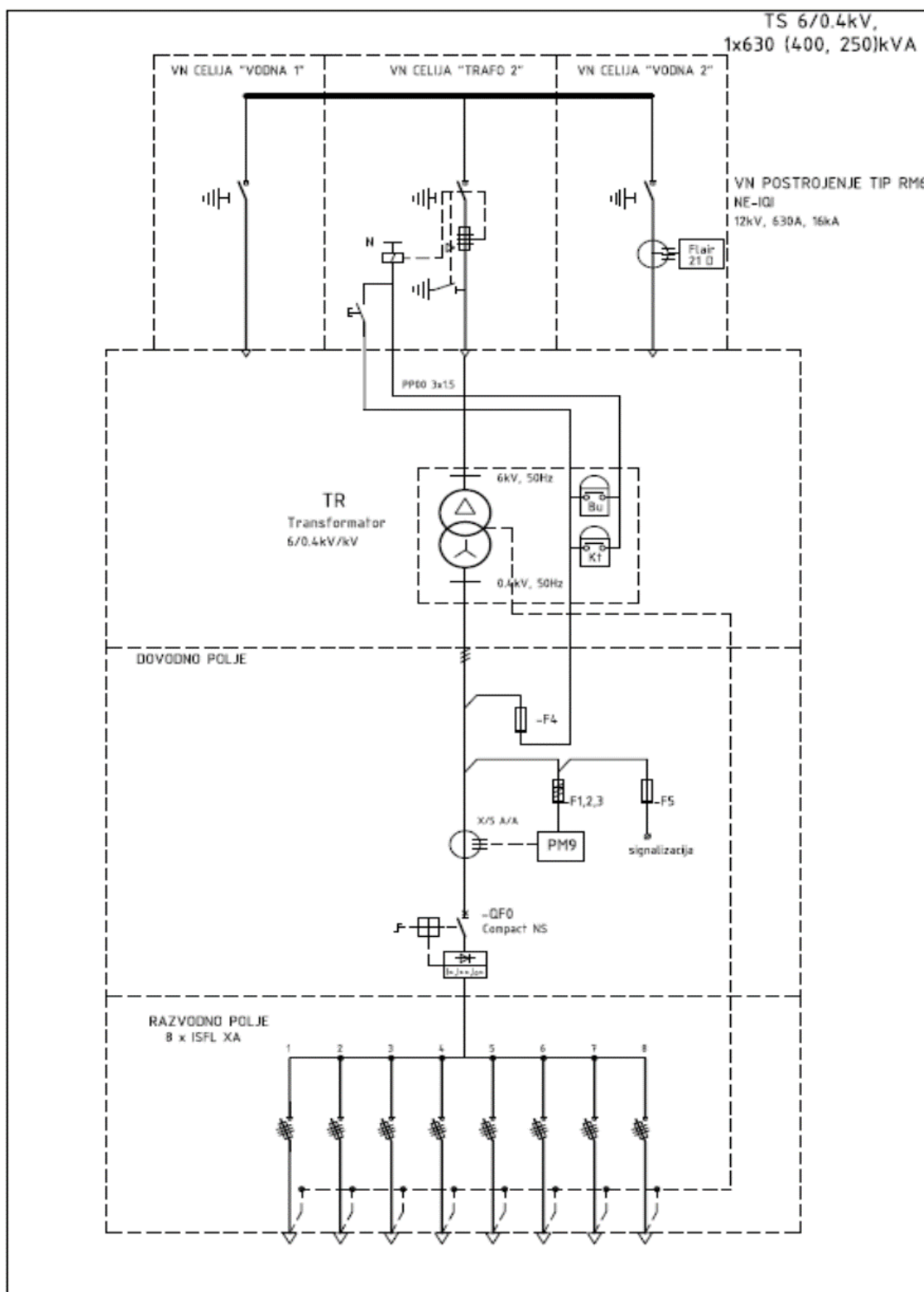
Једнополна шема ТС
