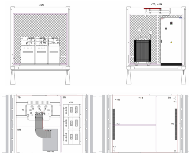
Слика 1. Позиција опреме у МЛТС
